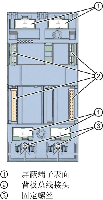
图 2-5 CPU 1516-3 PN/DP 的后视图
