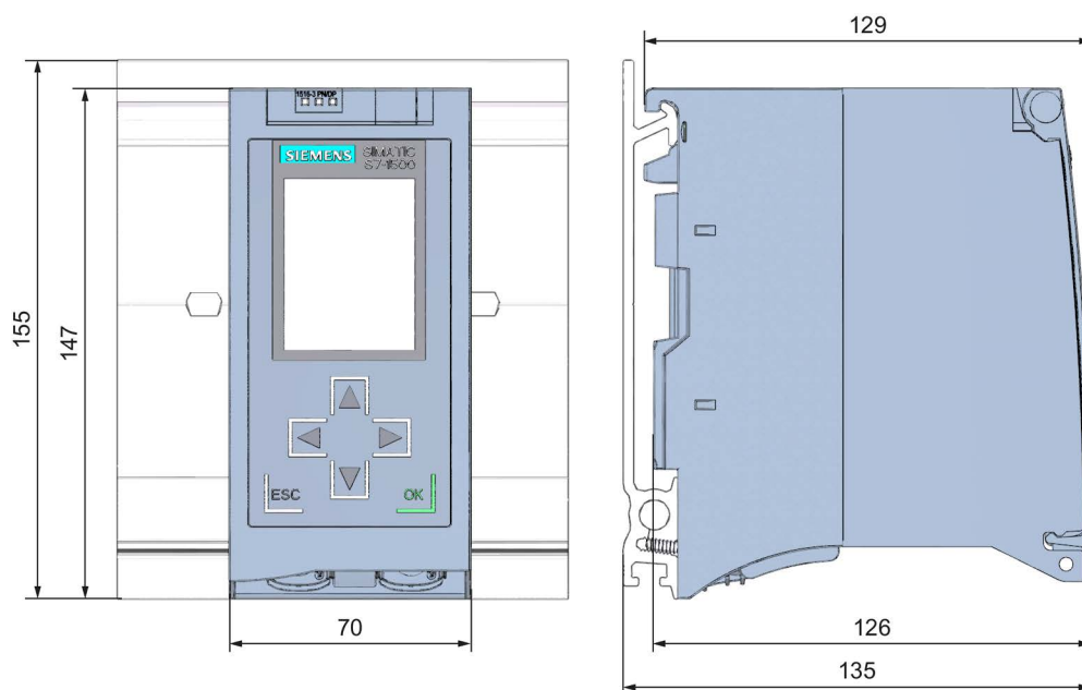
图 A-1 CPU 1516-3 PN/DP 的尺寸图，正视图和侧视图
