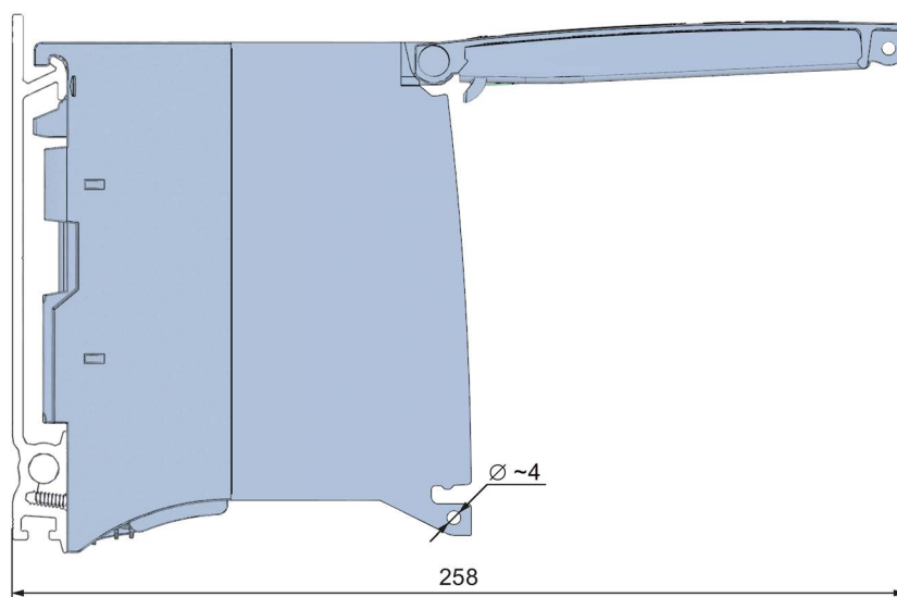
图 A-2 CPU 1516-3 PN/DP 的尺寸图，带有打开前盖的侧视图
